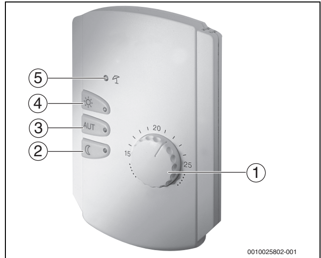
Res. 24 Uzaktan kumanda BFU
