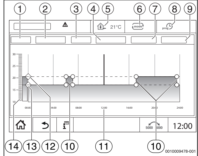
Res. 26 Zaman programı
