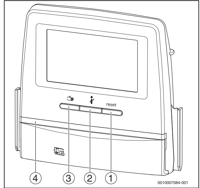
Res. 16 Fonksiyon tuşları
