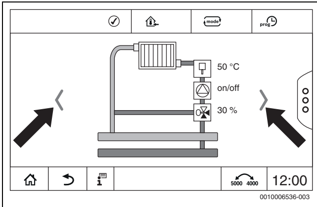
Res. 10 Ekranlar arası geçiş
