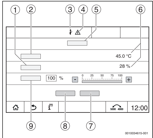
Res. 17 Atık gaz testi > Kazan ayarları göstergesi
