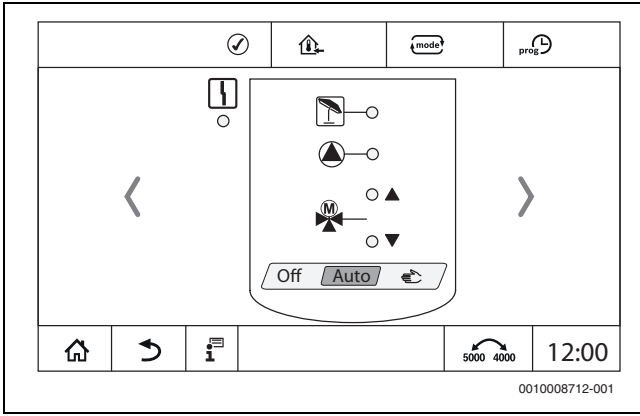
Res. 14 4000 serisi ısıtma devresi görünümü
